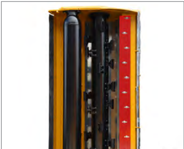
MU-Vario® für eine optimierte Einlass- und Gehäuseform und einen stufenlos wählbaren Zerkleinerungsgrad. Dadurch werden ideale Mulchqualität und Zerkfaserung erreicht.
