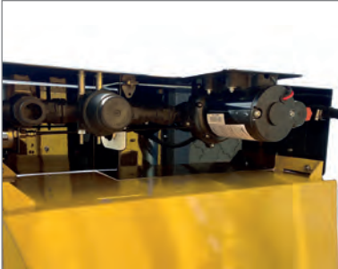
Pumpeneinheit bestehend aus Saugfilter, Elektropumpe, Druckfilter und Druckregelventil.
