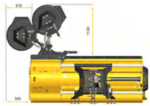
MU-FlexDisc 60 Hydraulische Mähzscheibe mit Wirkdurchmesser Ø 600 mm inkl. mechanischem Federzug (Ölbedarf max. 30 l/min).
