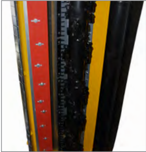
MU-Vario® für eine optimierte Einlass- und Gehäuseform und einen stufenlos wählbaren Zerkleinerungsgrad. Dadurch werden ideale Mulchqualität und Zerkleinerung erreicht.
