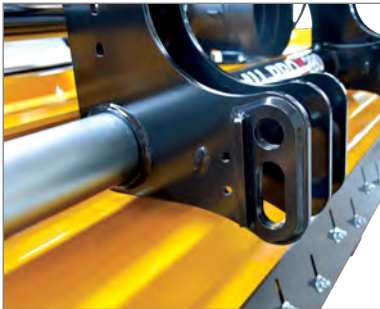
Langlöcher an den Ober- und Unterlenkeranbaupunkten ermöglichen zusammen mit der Schwenk-Stützwalze eine sehr gute Bodenanpassung.
