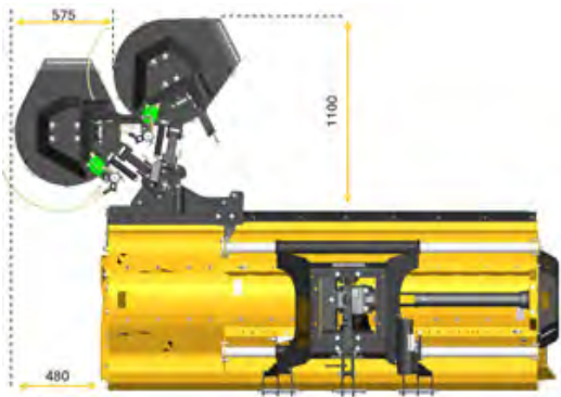
MU-FlexDisc 60 Plus Hydraulische Mähzscheibe mit Wirkdurchmesser Ø 600 mm inkl. hydraulischer Tastersteuerung (Ölbedarf max. 35 l/min).
