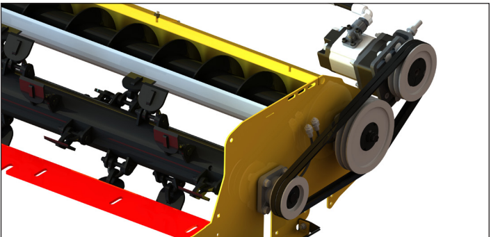
Keilriemen für sichere Kraftübertragung und Überlastsicherung.
